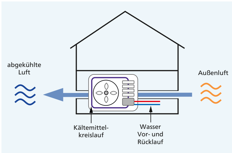
Abbildung 2.6 Innenaufstellung einer Luft-Wasser-Wärmepumpe in Monoblockbauweise
