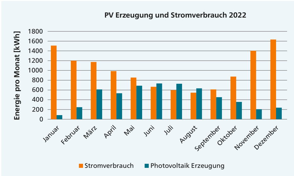
Abbildung 6.17 Stromverbrauch und PV-Ertrag nach Monaten
