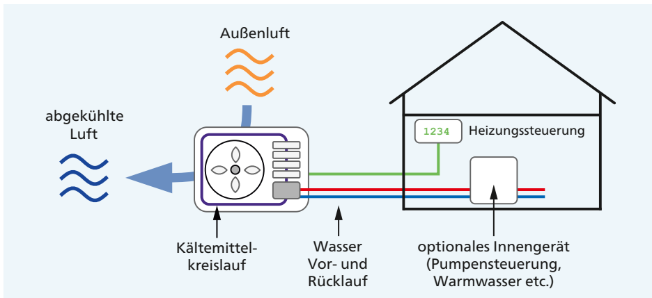
Abbildung 2.5 Schema einer Luft-Wasser-Wärmepumpe in Monoblock-Bauweise
