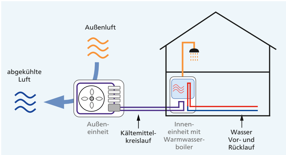
Abbildung 2.8 Luft-Wasser-Wärmepumpe in Splitbauweise mit integriertem Warmwasserboiler
