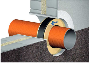
Abb. 4.3-14 Rohrdurchdringung mit Klebeflansch und Dichtungsring
