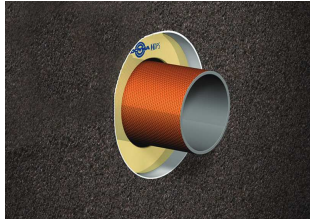
Abb. 4.3-15 Fertige Rohrdurchdringung in einer Kelleraußenwand
