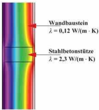
Abb. 1.4: Eindimensionale Wärmebrücke
