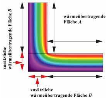
Abb. 1.5: Zweidimensionale Wärmebrücke
