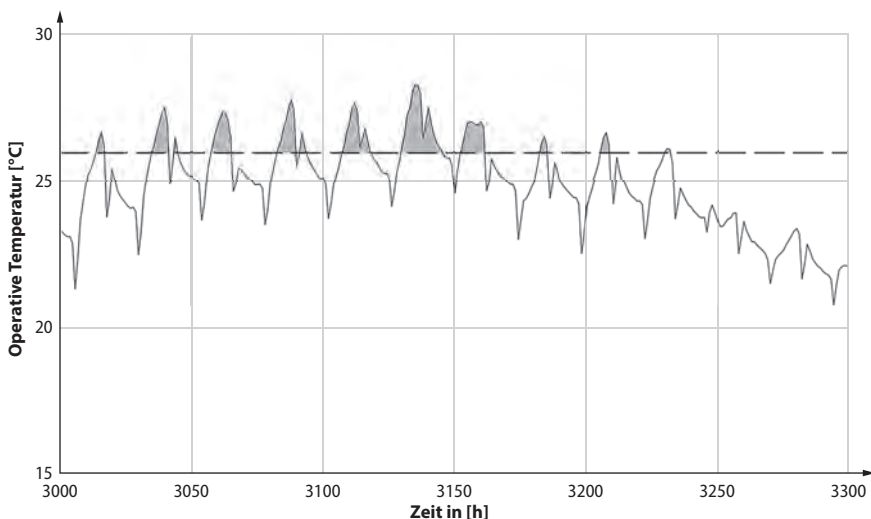
Bild 18. Graue Integralfäche der Übertemperaturgradstunden über 26 °C im Zeitraum 3000 bis 3300 Stunden eines Jahres [4]
