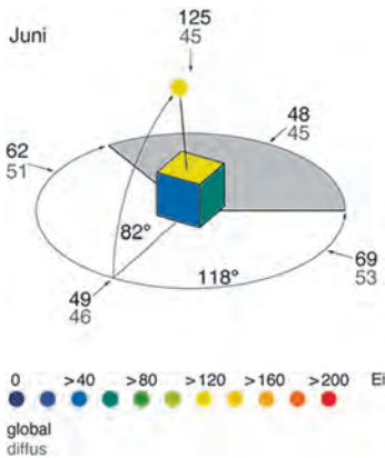
Bild 3. Visualisierung der auftretenden Strahlung auf der Oberfläche in kWh/(m 2 Monat) mittels Farbcodierung [29]
