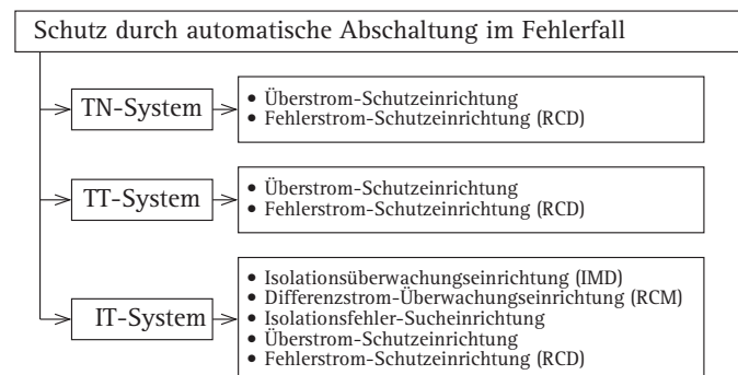
Bild 5.2 Schutzmaßnahmen für den „Schutz durch automatische Abschaltung im Fehlerfall“ in den verschiedenen Netzsystemen
